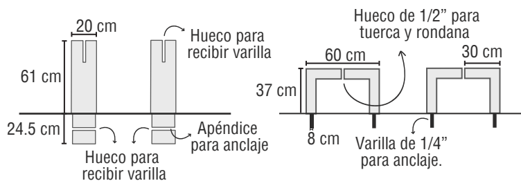
Base de mesa. Sección transversal.
