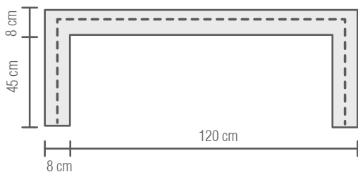
Sección longitudinal
