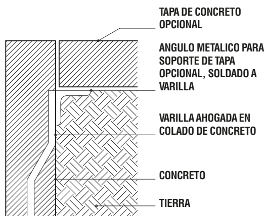
DETALLE 5 (CON TAPADERA) ESCALA 1:20
