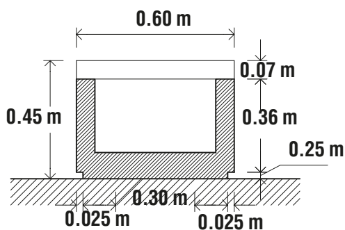
5 SECCION 5 NP02 ESCALA 1:20
