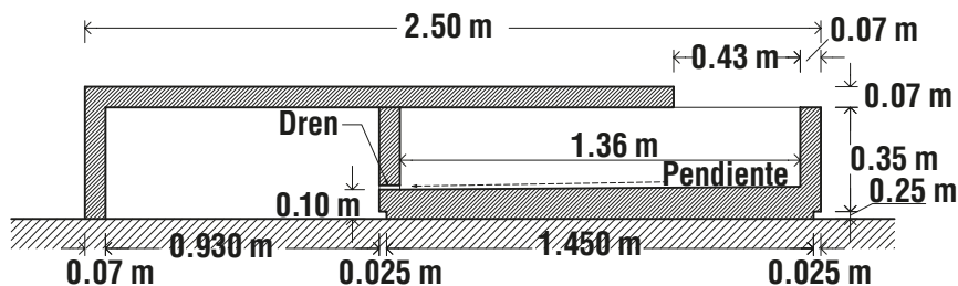
3 NP01 SECCION 3 ESCALA 1:20
