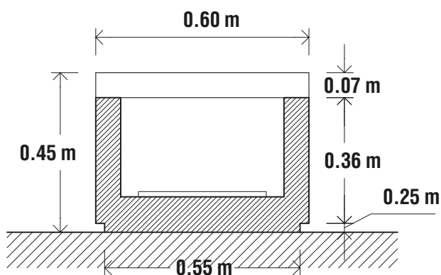
5 NP01 SECCION 5 ESCALA 1:20
