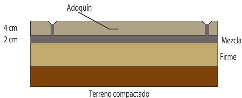
croquis esquemático
