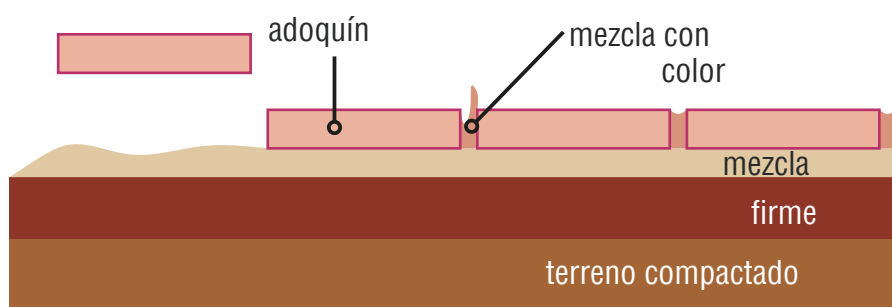
croquis esquemático
