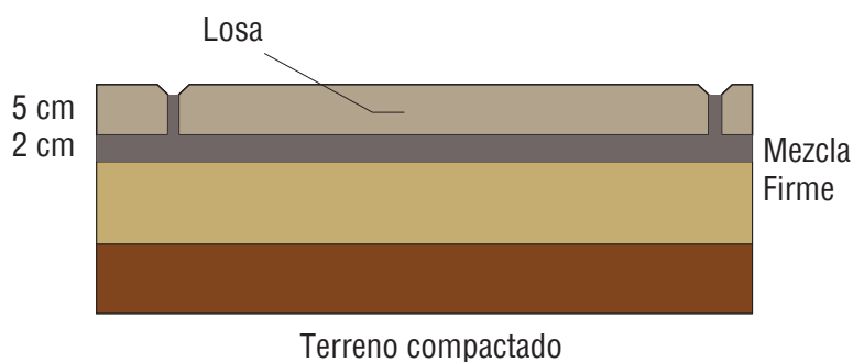
croquis esquemático
