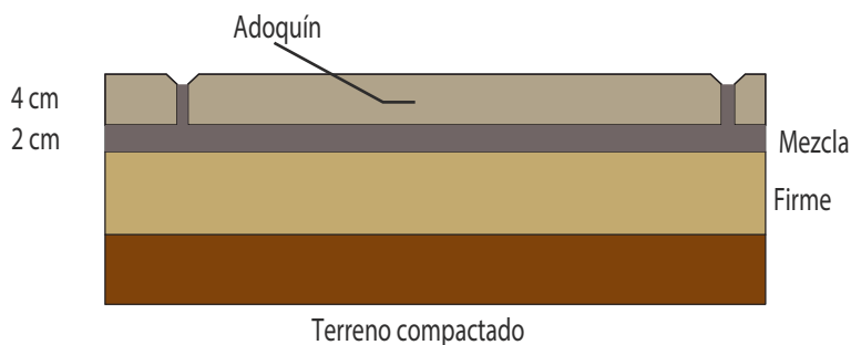
croquis esquemático
