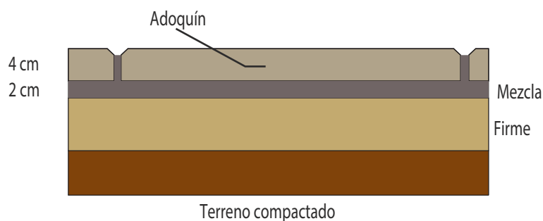
croquis esquemático
